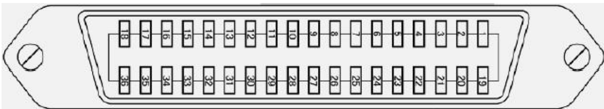
HANDLER 接口引脚图
